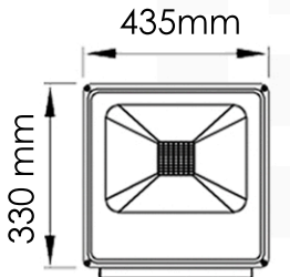
ALZADO FRONTAL
