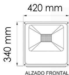
ALZADO FRONTAL
