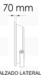
ALZADO LATERAL
