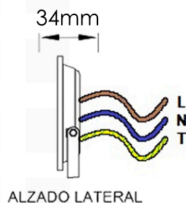
ALZADO LATERAL
