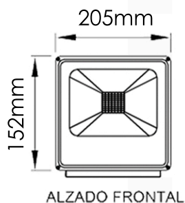
ALZADO FRONTAL
